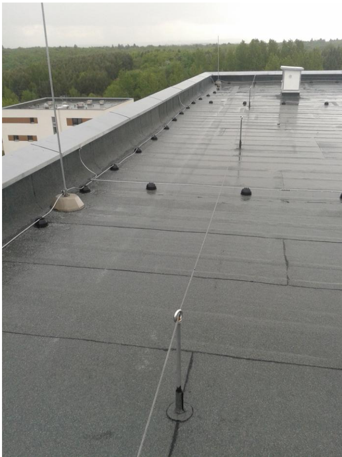
Systémy pro prevenci pádu ze střechy
